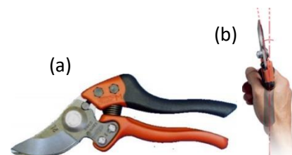
Sécateur ergonomique inclinaison verticale (a) et latérale (b) de la tête de coupe
